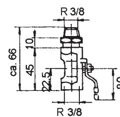
Dräneringsventil 16/30
